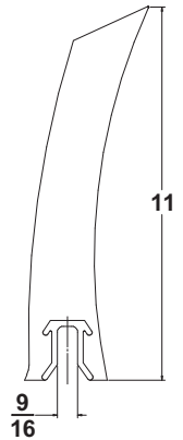
E11 Series Blade Profile (Scale 1.5:1)
